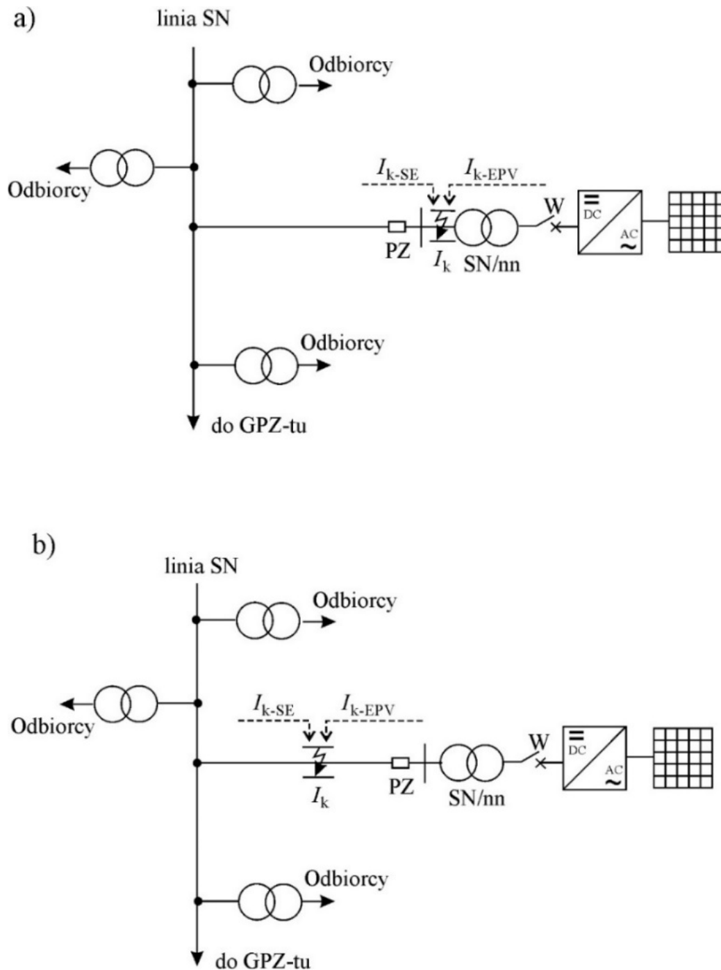
Rys. 15.2.7. Zjawiska podczas zwarcí międzyfazowych dla EPV przyłączonej do linii SN
