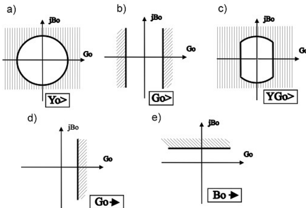
Rys. 13.3.3. Charakterystyki zabezpieczeń ziemnozwarciowych
